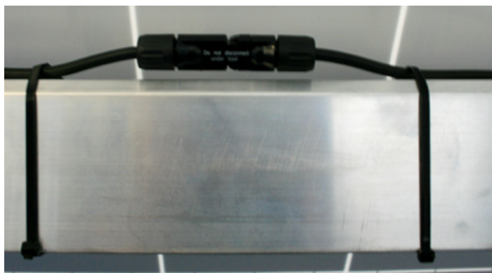
図11: 架台レールから離して固定することで、空気循環や排水が確保されたコネクタのベストプラクティスな設置が可能
