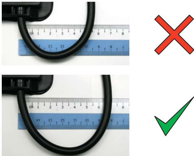
図8: 既存のジャンクションボックスでのケーブルの正しい曲げと間違った曲げの例
